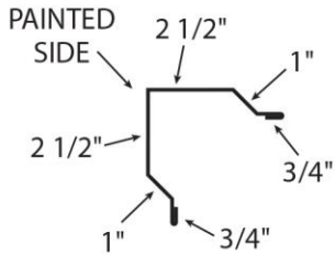
MINI RAKE
