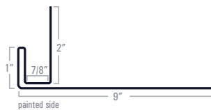
Overhead Door Jamb
