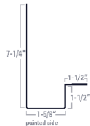
DJ8 JAMB TRIM
