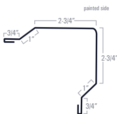
Mini Corner/Rake
